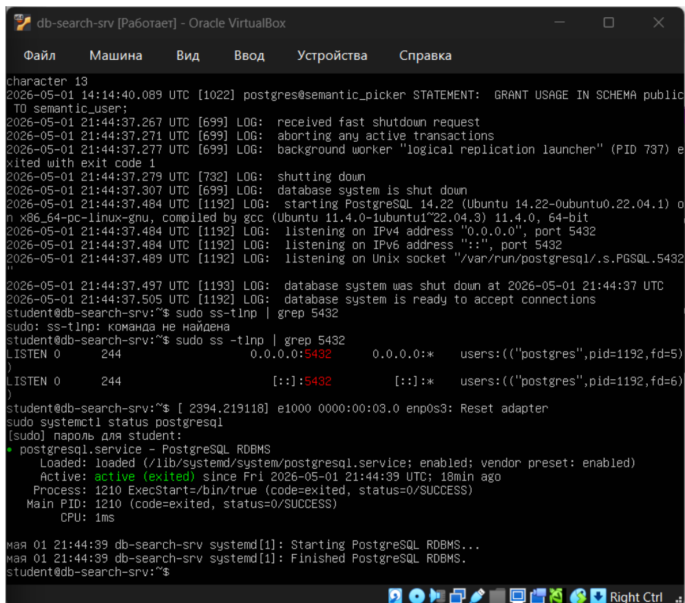
Рисунок 15 - Работающий PostgreSQL
